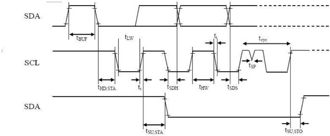
图 1、双线通讯交流参数图
