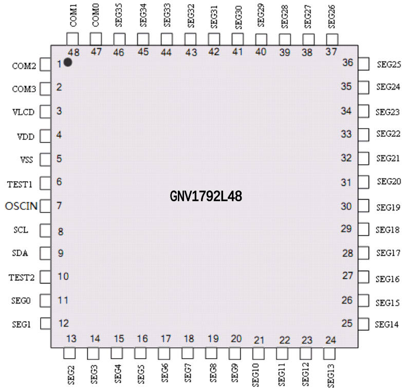
LQFP48
