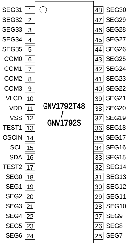
TSSOP48/SSOP48
