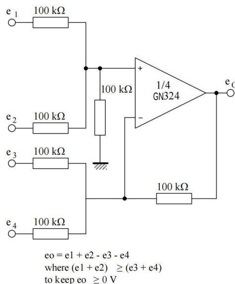
图4、直流加法放大器
